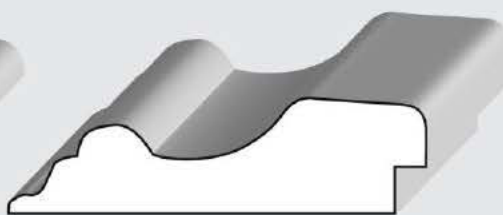
AB 512 3/8" x 2-3/8"
